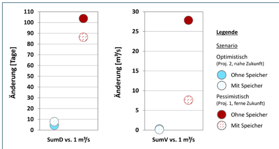
Abb. 6: Absolute Änderung der Anzahl an Tagen im Wasserhaushaltsjahr, an denen der Grenzwert von 1 m 3 /s am Pegel Hof unterschritten wird (SumD) sowie das daraus resultierende Defizit SumV – Darstellung je für das optimistische und pessimistische Teilszenario mit und ohne Speicher.
